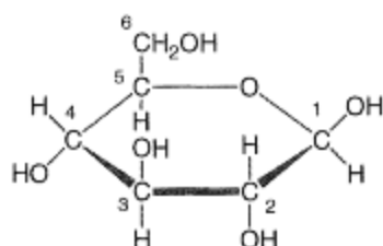
図1 グルコースの環状構造の1つ
