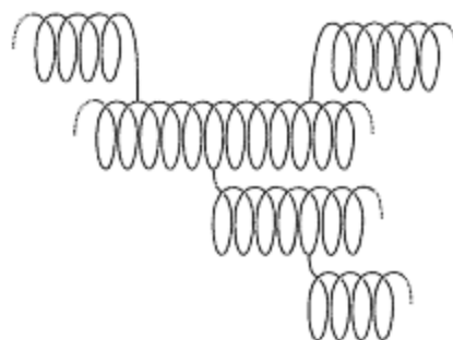
図3 〔ウ〕の枝分かれ構造の模式図
