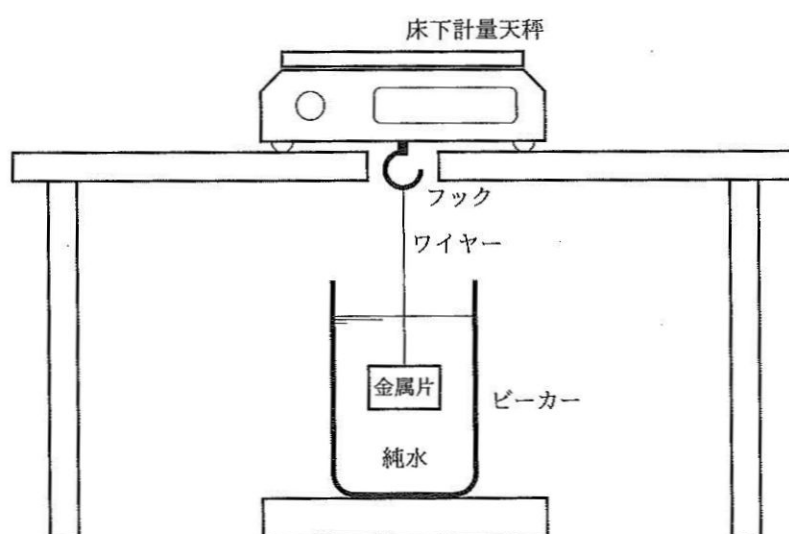
図 実験装置
